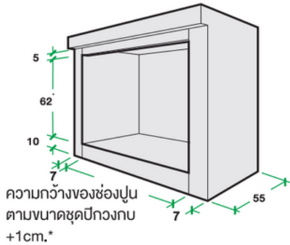
ภาพด้านหน้าช่องเคาน์เตอร์ปกติ
