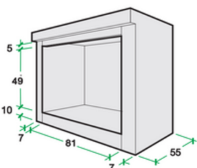
ภาพด้านหน้าช่องเคาน์เตอร์เตาแบบตั้งบนท็อป
